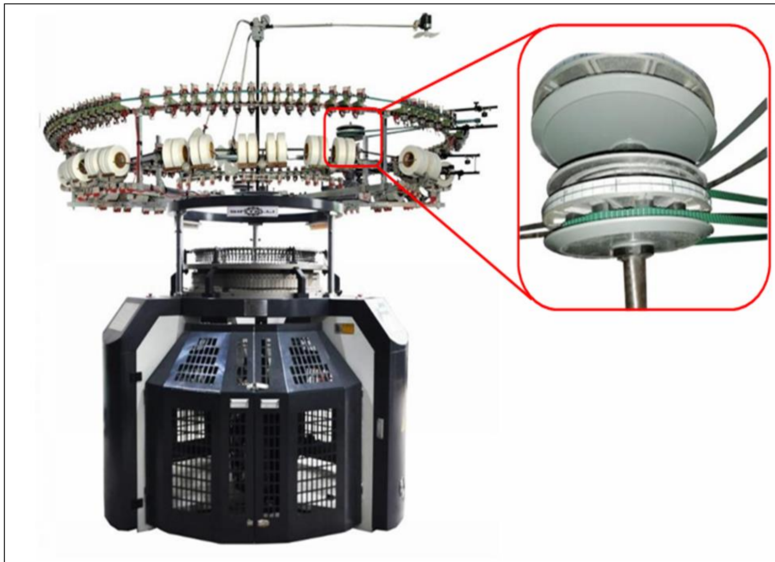
VDQ PULLEY
